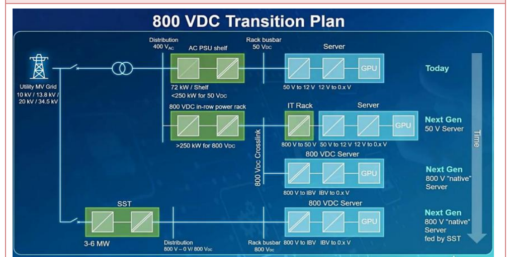
圖 2：伺服器電源架構
